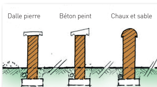
Principes de couronnements © CAUE 44
